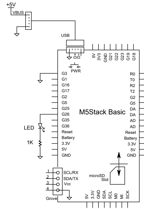
M5Stack Basic Lチカ 電気回路図
